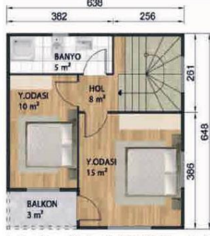
1. Kat Planı 38m 2 + 3m 2 BALKON = 41m 2
