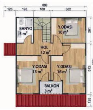
1. Kat Planı 56m² + 3m² BALKON = 59m²
